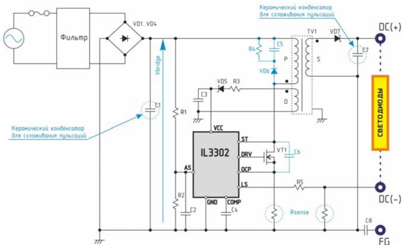
Рисунок 24 – Типовая схема применения микросхемы IL3302
