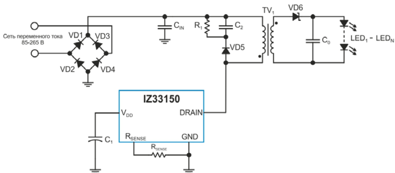
Рисунок 35 – Типовая схема применения микросхемы IZ33150 с изолированным выходом
