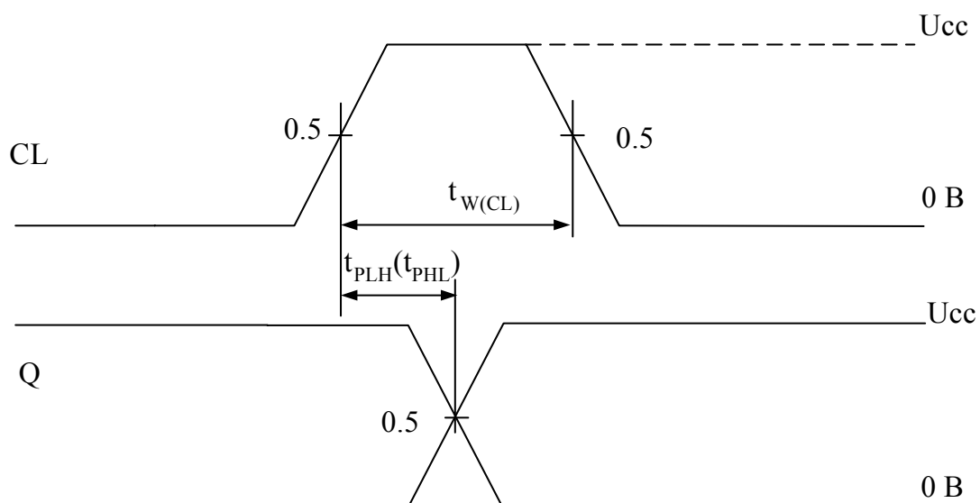
Рисунок 1 – Временная диаграмма работы микросхемы
